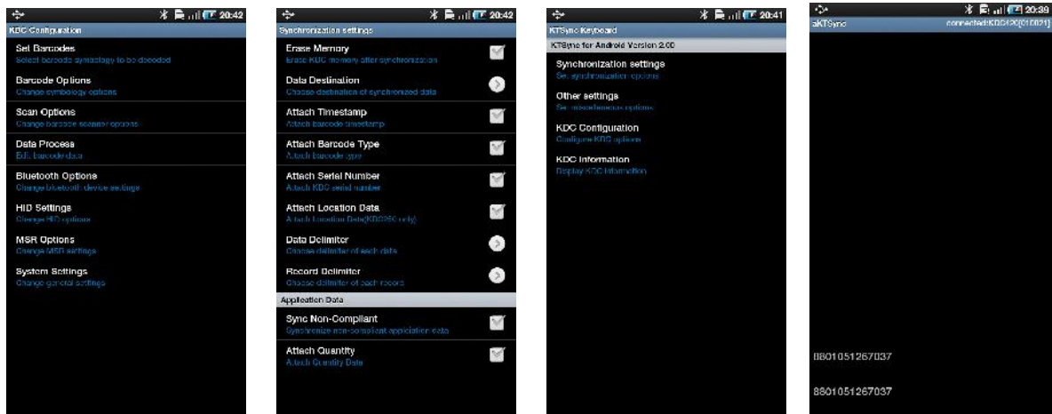
그림 18 – Android aKTSync
