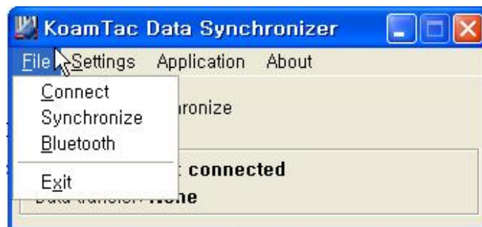
그림 8 - File Menu
