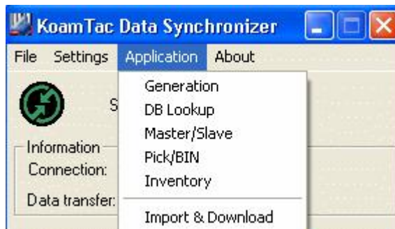
그림 10 - Application Menu
