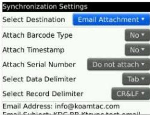
그림 20 - Blackberry bKTSync
