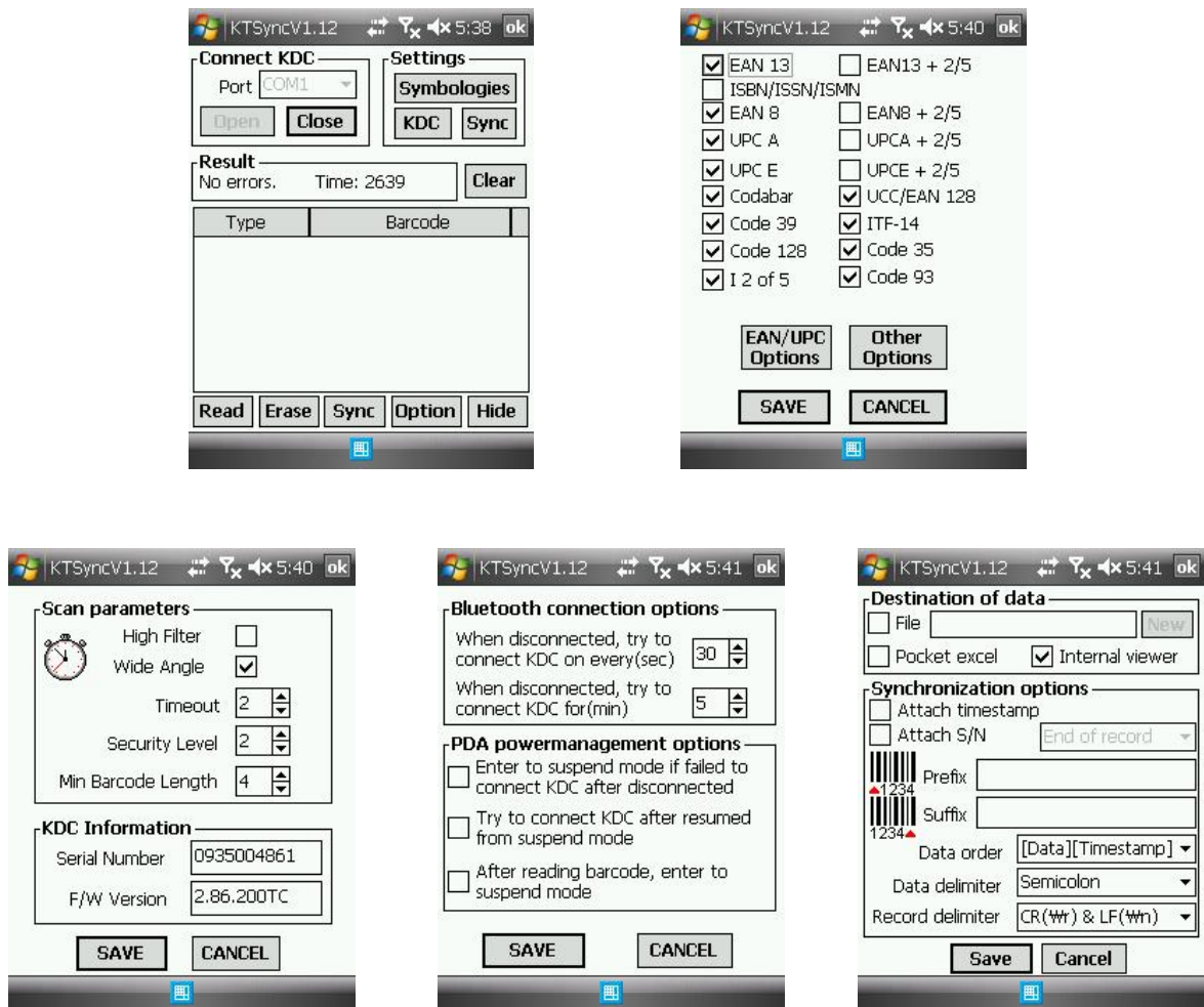
그림 17 – Mobile pKTSync
