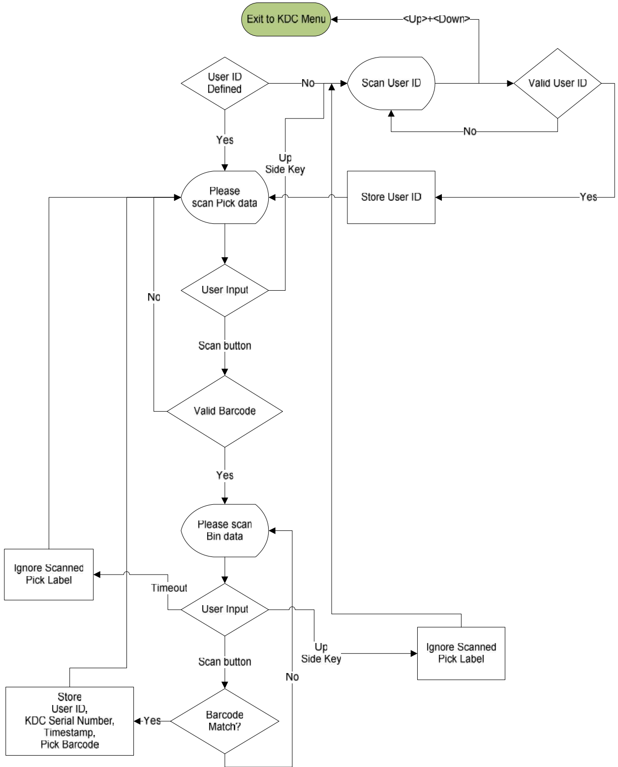
그림 28 - Pick/BIN Application Flow Chart
