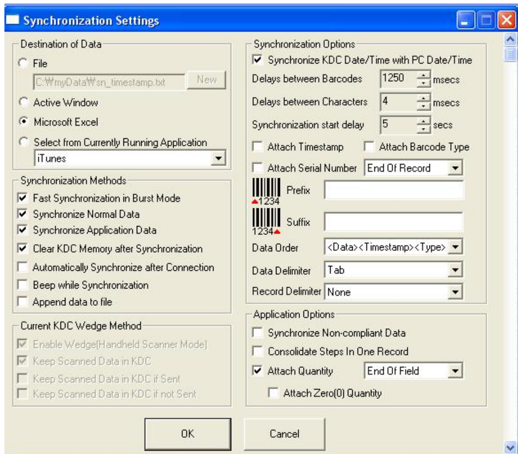
그림 14 - KTSync® Synchronization Settings
